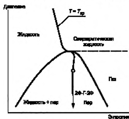
б) Для переходных вариантов от «регулярных» сред к «ретроградным» средам, с k = c_p/c_v , близким к 1,1
