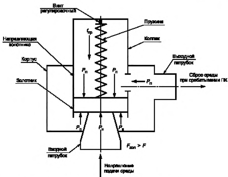
Рисунок В.1 — Статические давления в типовом неразгруженном двухпозиционном ПК
