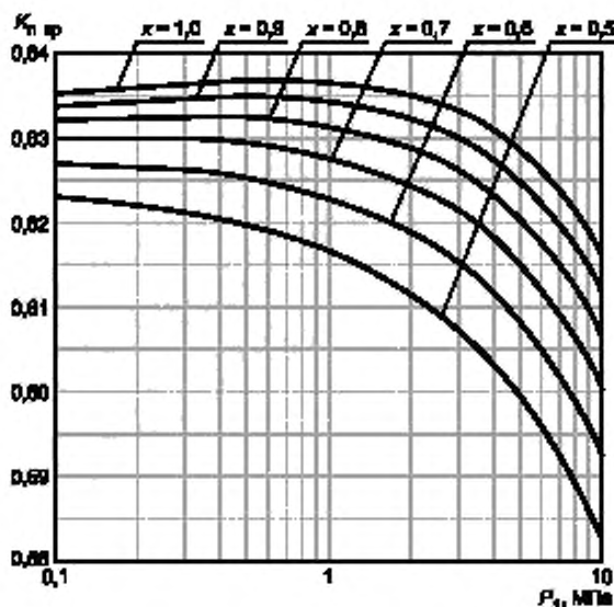
Рисунок Е.9 — Зависимость K_{кр} = f(P_1) для влажного водяного пара
