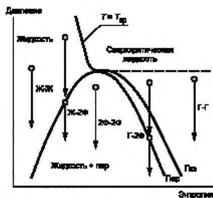
а) Для «регулярных» сред, с k = c_p/c_v > 1,1
