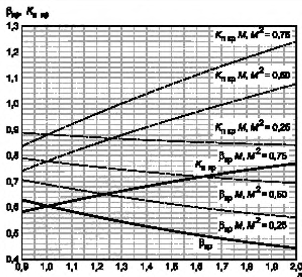
Рисунок Е.2 — Коэффициенты \beta_{кр} и K_{n,кр} для уравнения постоянного показателя изоэнтропы
