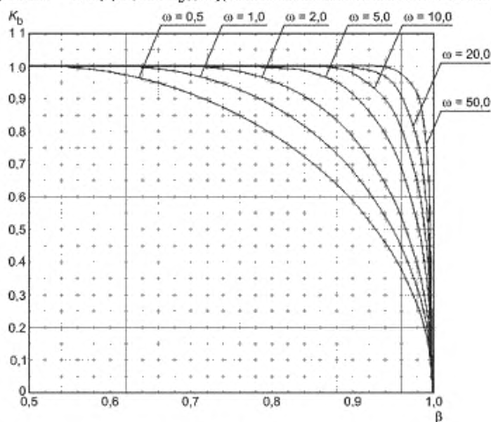
Рисунок Е.6 — Коэффициент K_b для омега-метода
