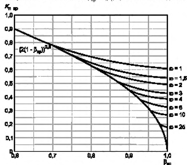
Рисунок Е.8 — Зависимость K_{n\text{кр}} = f(\beta_{кр}) при вскипании жидкости
