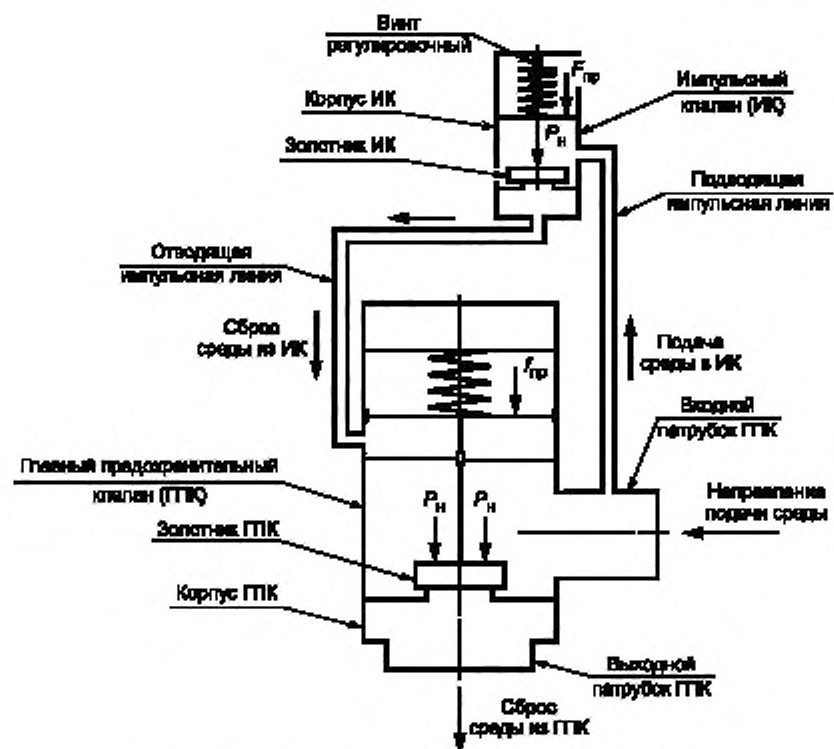
Рисунок В.3 — Импульсно-предохранительное устройство
