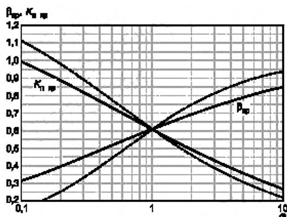
Рисунок Е.3 — Коэффициенты \beta_{\omega} и K_{1\omega} для омега-метода
