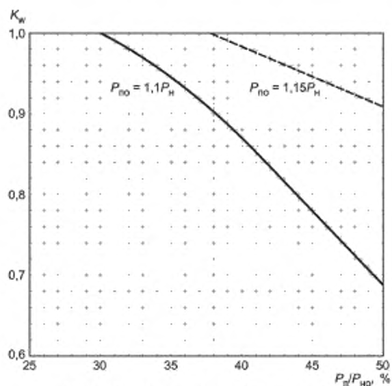
а) При работе клапанов на газообразных средах
