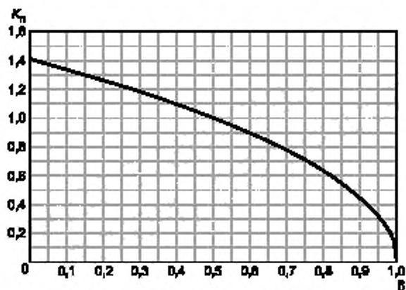
Рисунок Е.1 — Коэффициент K_n для несжимаемой жидкости
