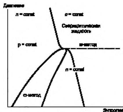
а) Для ретроградных сред, \omega и k = \rho_p/\rho_r близки к 1,0
