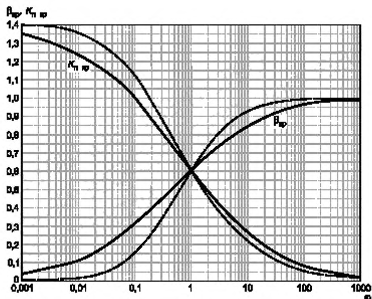
Рисунок Е.3 — Коэффициенты \beta_{\omega} и K_{1\omega} для омега-метода
